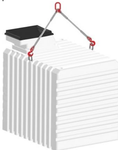
Рисунок 3. Крепление стропой СТП-1.
