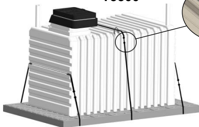
Рисунок 5. Схемы якорения погребов.
