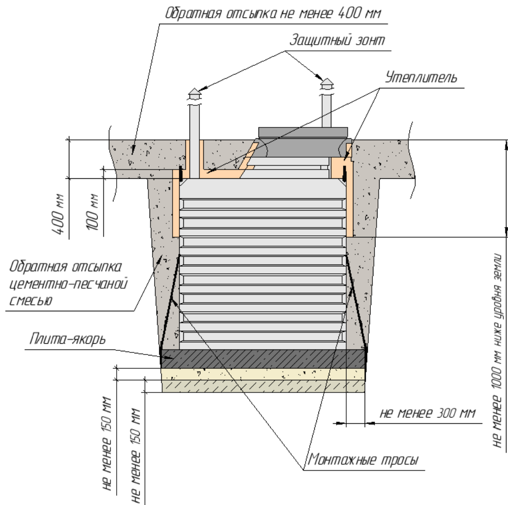
Схема монтажа погреба Т3500 с нижним якорением
