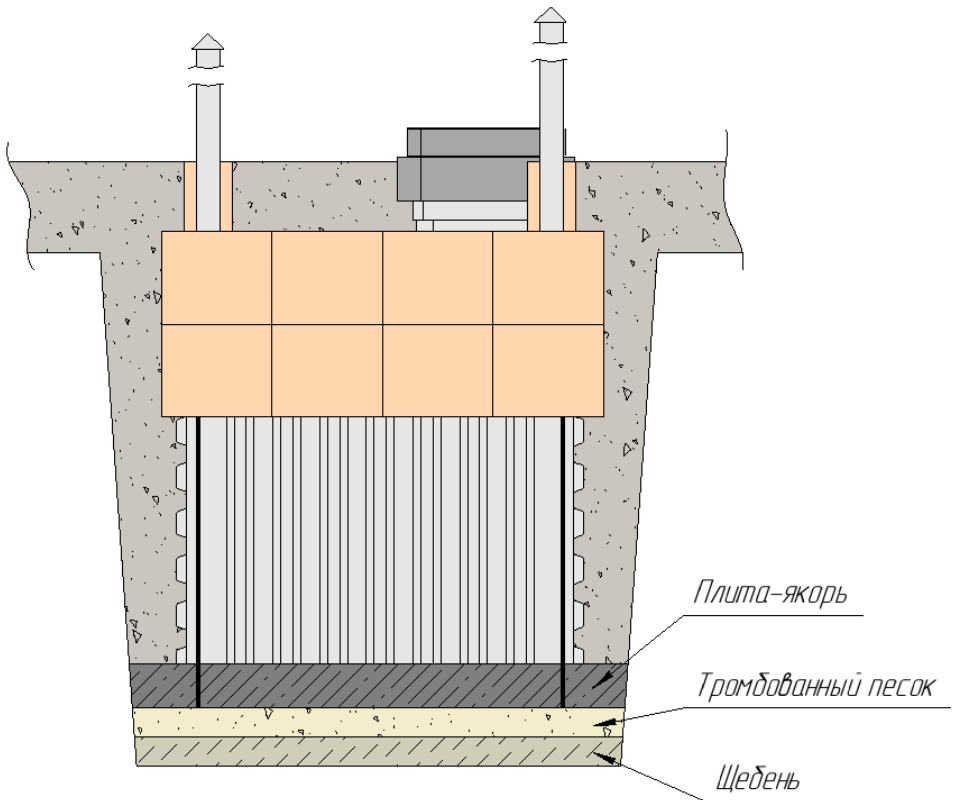
Схема монтажа погреба Т1500-3000 с нижним якорением
