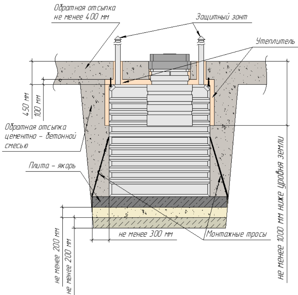
Схема монтажа погребов Т1900-К, Т2500-К с нижним якорением
